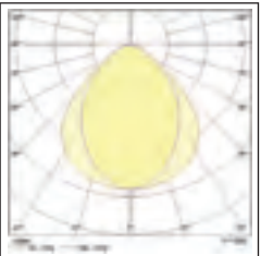
T8 - 2 x 58W
